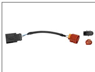
7.53520 - Adapterkabel ersetzt Pierburg: 4.07360.52.0
