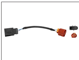
7.53520 - Câble d'adaptateur remplace Pierburg : 4.07360.52.0
