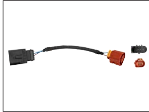
7.53520 - كابل مهائيء يحل محل PIERBURG: 4.07360.52.0
