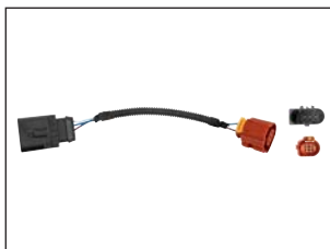
7.53520 - Cavo adattatore sostituisce Pierburg: 4.07360.52.0
