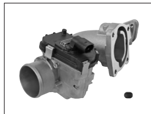
7.53640 - Корпус дросселя заменяет Pierburg : 7.03703.49.0
