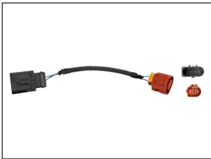
7.53520 - Cable adaptador reemplaza a Pierburg: 4.07360.52.0
