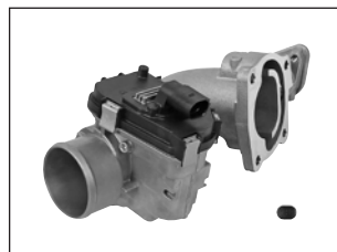
7.53640 - Boîtier papillon remplace Pierburg : 7.03754.09.0
