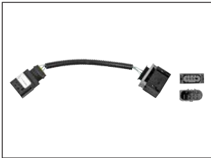
7.53630 - Cable adaptador reemplaza a Pierburg: 4.07360.49.0
